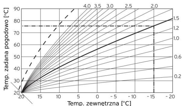
Krzywe grzewcze obiegu.
